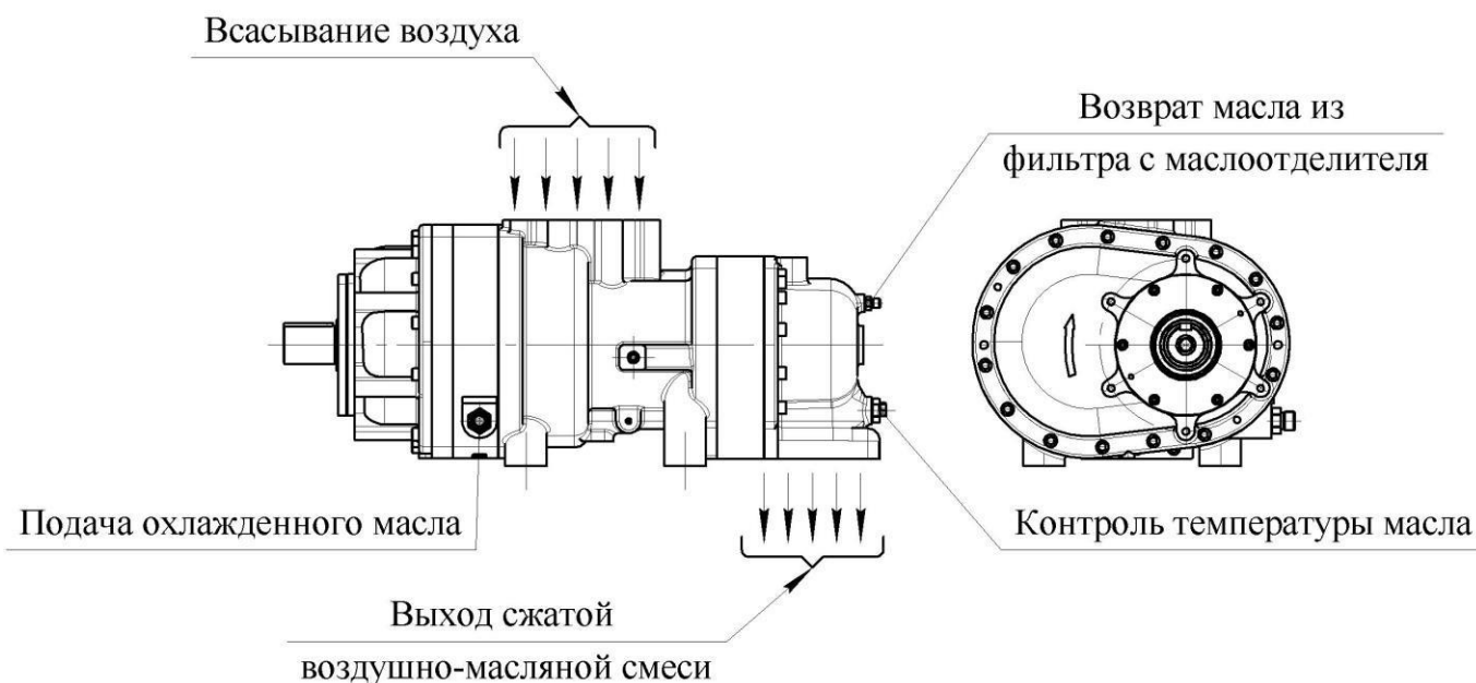
Общий вид блока винтового SCA20GRM:
