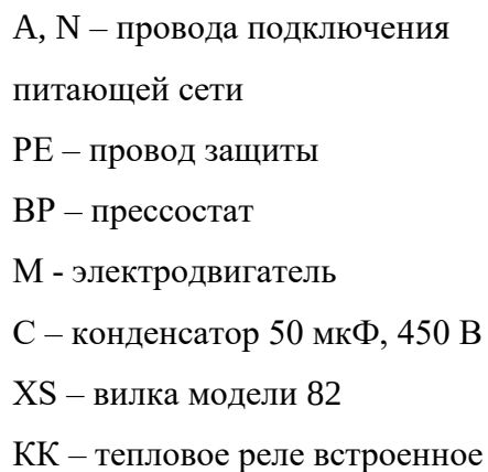
Рисунок А.1 - Схема электрическая принципиальная компрессора
