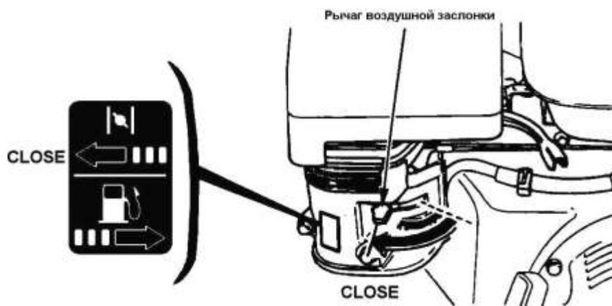
(рисунок 4). Не закрывайте воздушную заслонку, если двигатель горячий. Рисунок 4 – Рычаг воздушной заслонки в положении "CLOSE" ("Закрыто")
