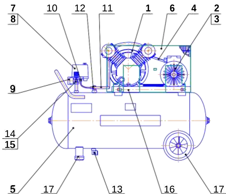
Рисунок 5 - Общий вид компрессора СБ4/С-100.LB24A
