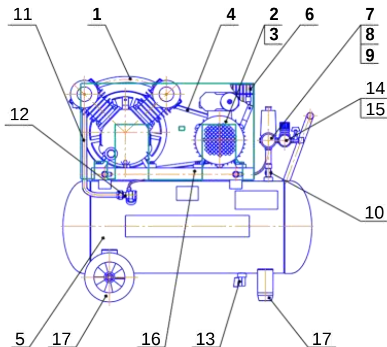
Рисунок 4 - Общий вид компрессора СБ4/С-50.LB24A
